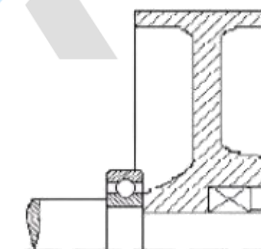
Fixação do volante
