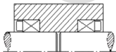
Acoplamento entre eixos
