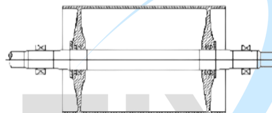
Fixação de tambores para transportadoras de correia
